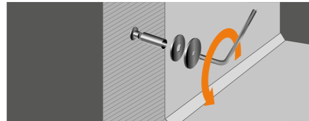
Schutzkappe mit einem 8er-Inbusschlüssel entfernen.
