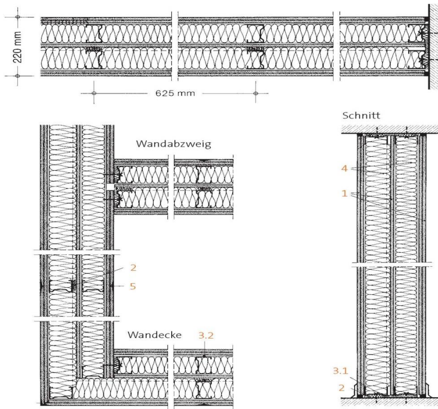
Abbildung 11: Trockenbausystem MW221RB/MW221RF
