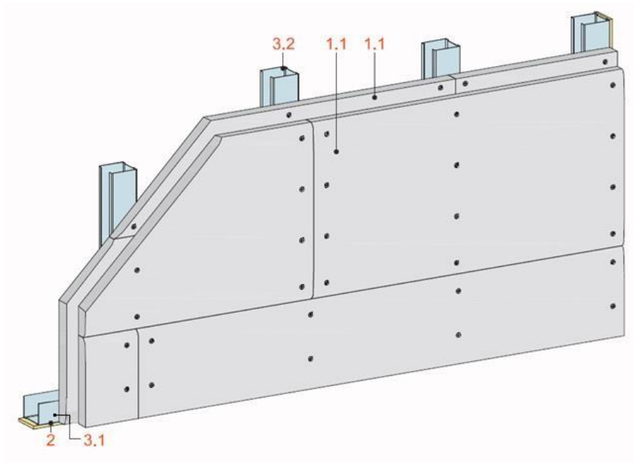
Abbildung 12: Trockenbausystem SW02DD/SW12DD
