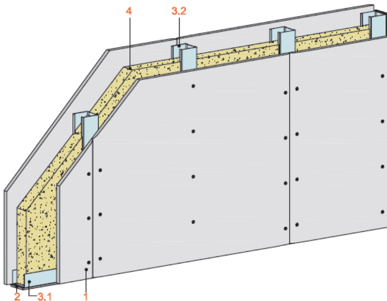
Abbildung 1: Trockenbausystem MW11RB/MW11RF/MW11DL
